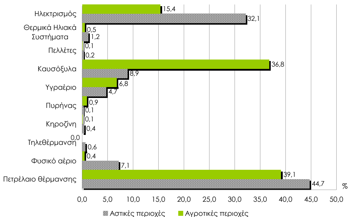
Γράφημα 5. Ποσοστιαία κατανομή (%) της συνολικής κατανάλωσης ενέργειας κατά τύπο καυσίμου και βαθμό αστικότητας
